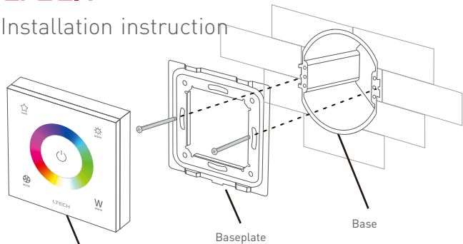
Baseplate
